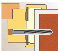
Montáž za pomoci pěny a šroubu do zdi
