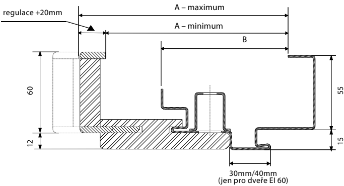
OBRÁZEK ŘEZU ZÁRUBNĚ PROJEKT
