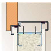
Zárubeň kątowa duża montaż na ścianie kartonowo-gipsowej
