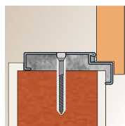
OPÁL Montáž s pomocí kotev
