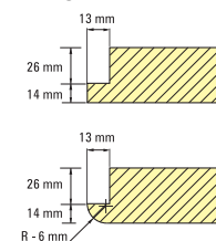
PROFIL HRANY
