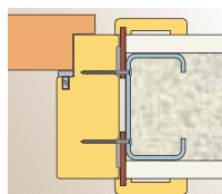
Montáž za pomoci šroubů do sádkartónové zdi
