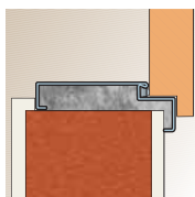
AGÁT Montáž bez dodatečných kotvících elementů.
