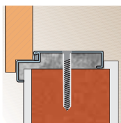
Montáž velké rohové zárubně do zdi nad 100 mm
