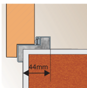
Montáž malé rohové zárubně
