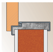
Montáž velké rohové zárubně do zdi 100 mm
