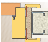
Montáž za pomoci pěny do sádkartónové zdi
