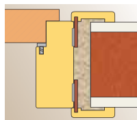
Montáž za pomoci pěny a šroubu do zdi
